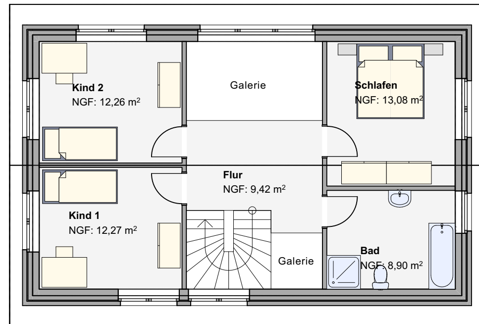
Dachgeschoss
