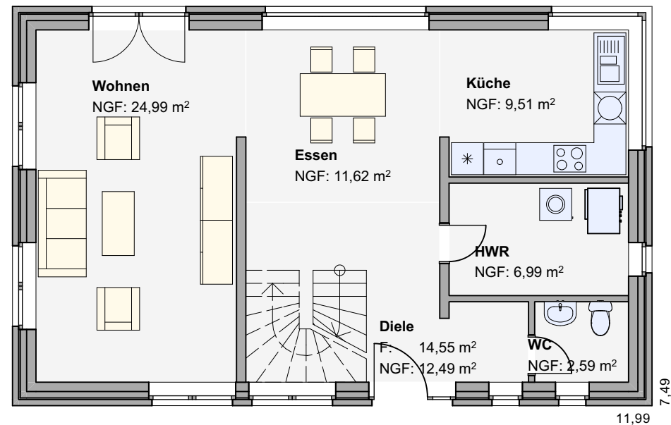
Erdgeschoss
