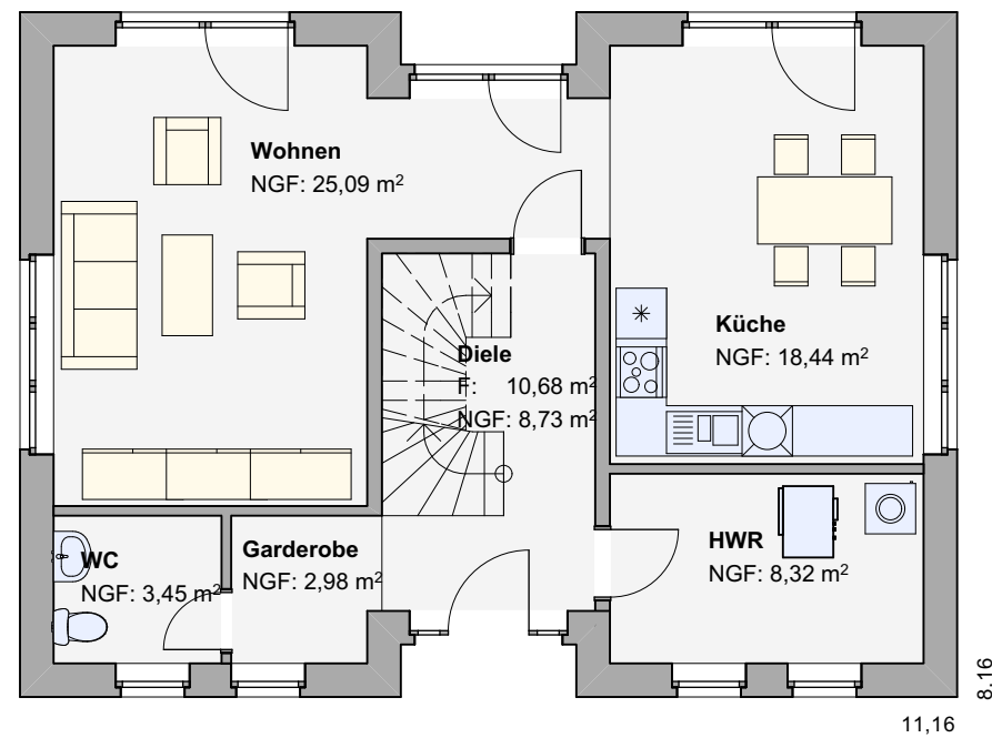
Erdgeschoss
