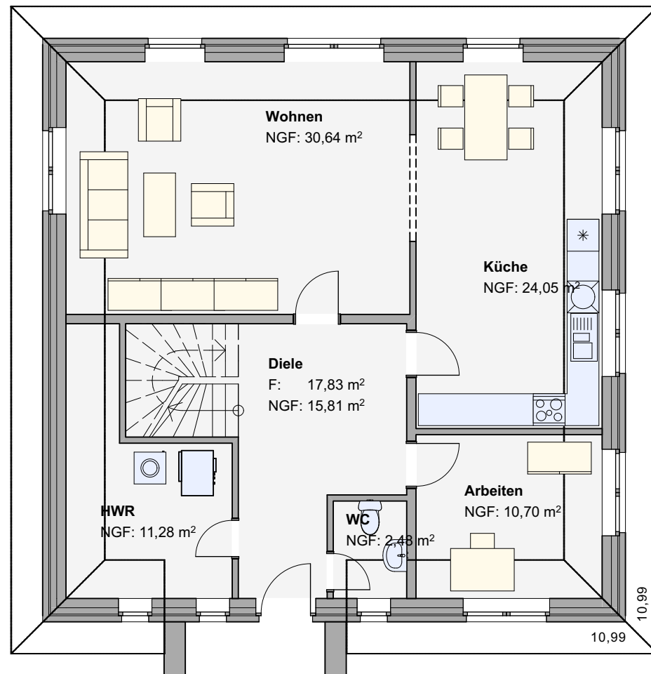
Erdgeschoss
