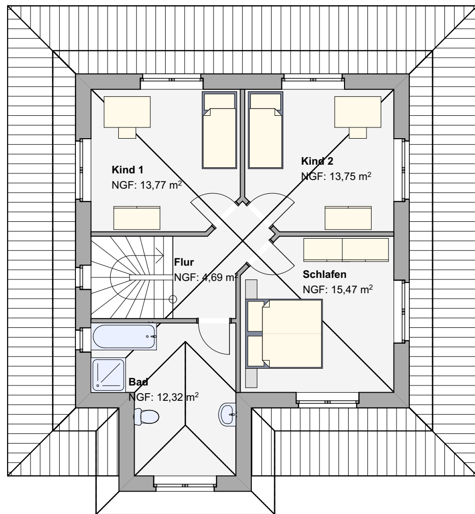
Obergeschoss
