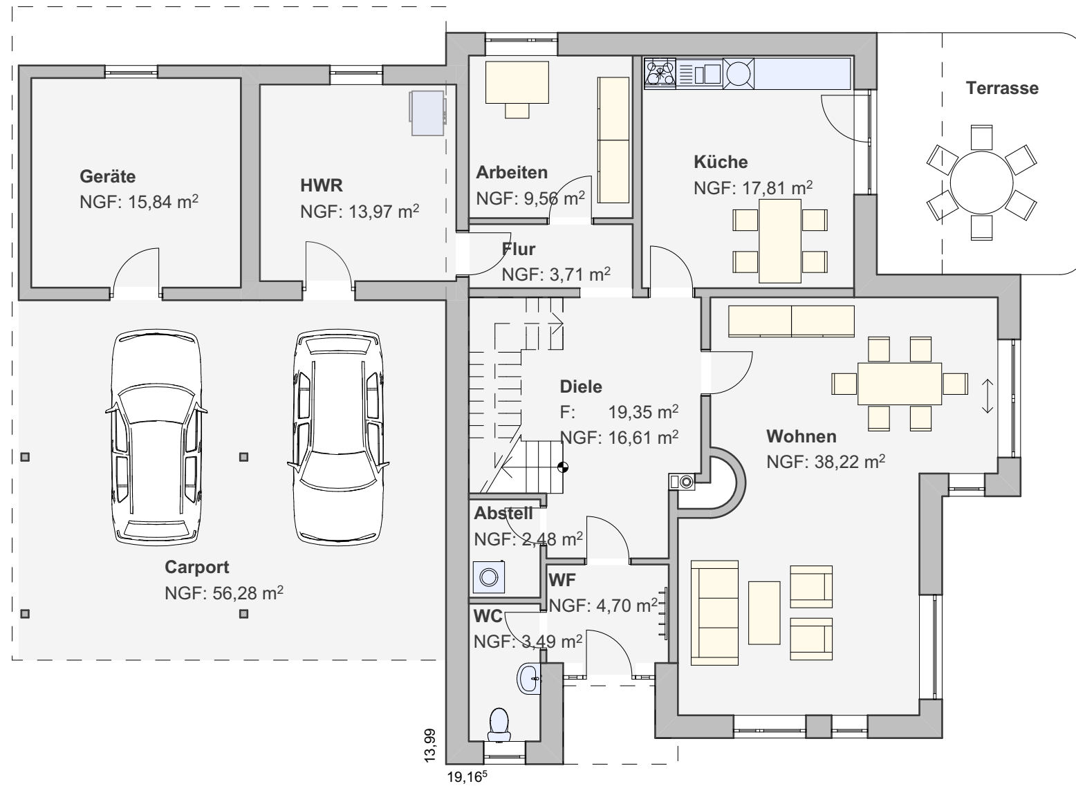
Erdgeschoss
