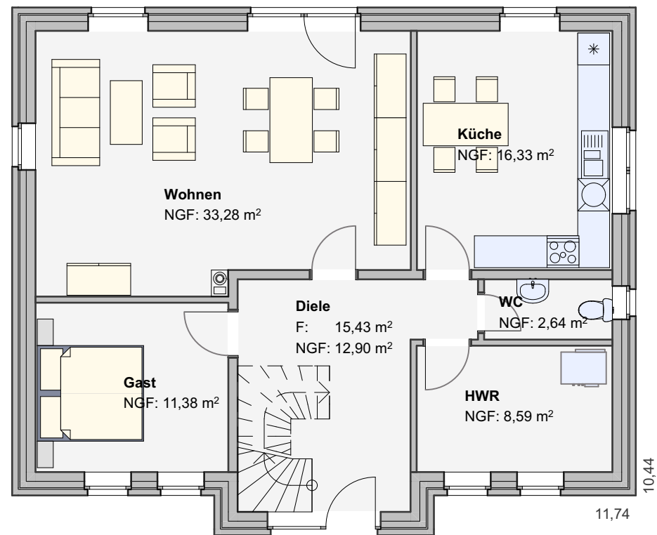
Erdgeschoss
