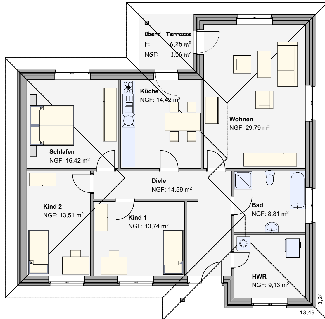
Erdgeschoss
