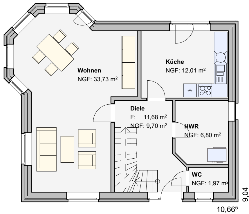
Erdgeschoss
