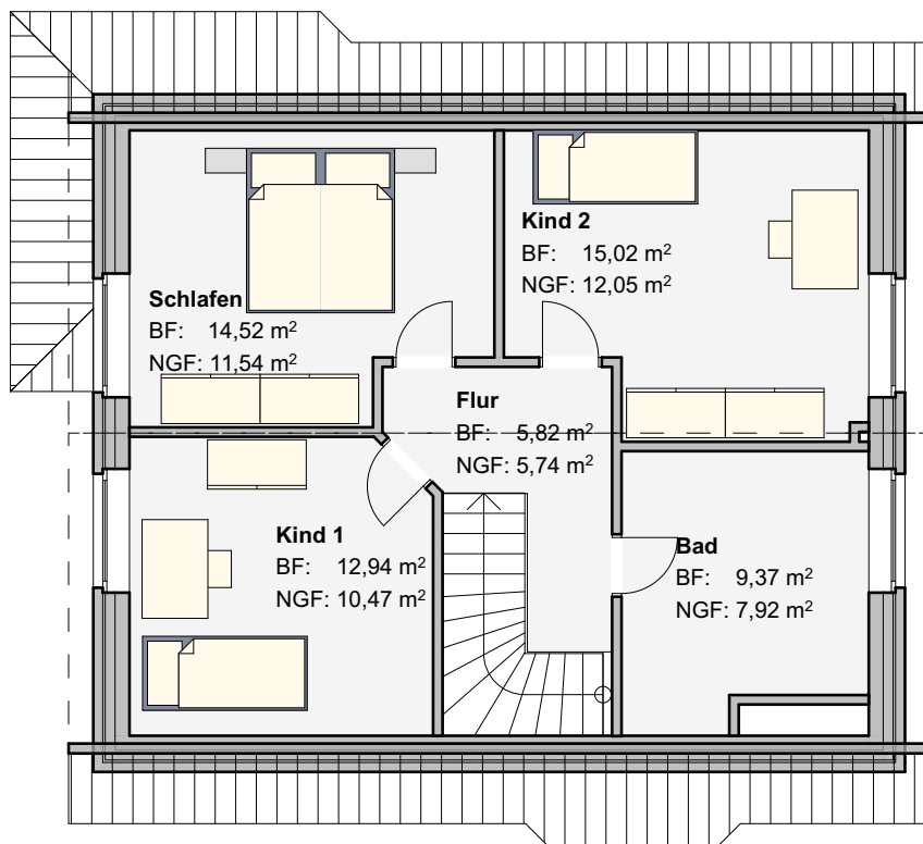
Dachgeschoss
