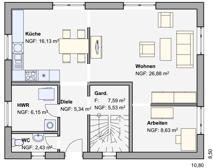
Erdgeschoss
