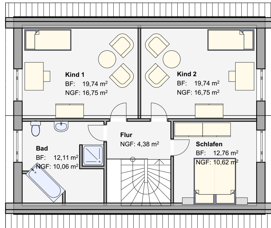
Dachgeschoss
