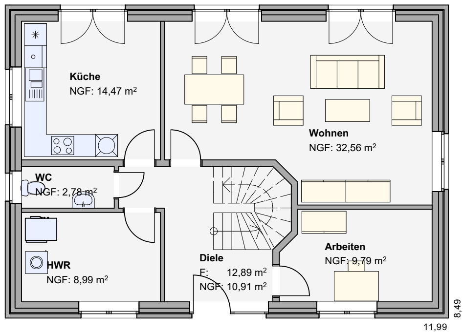
Erdgeschoss
