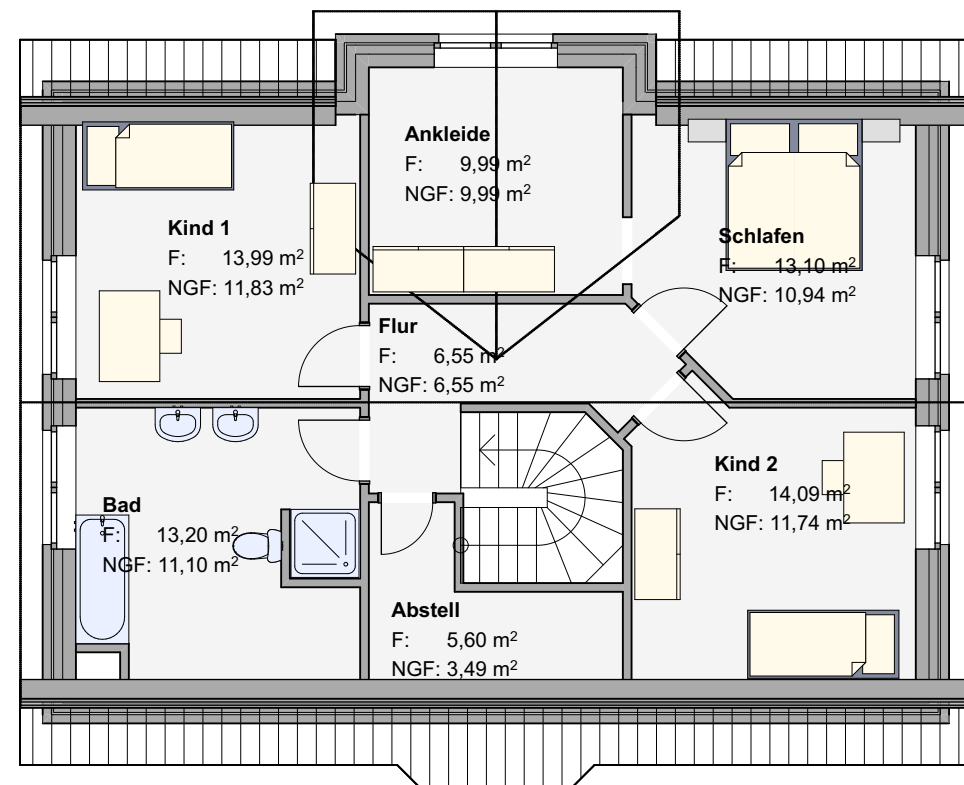
Dachgeschoss
